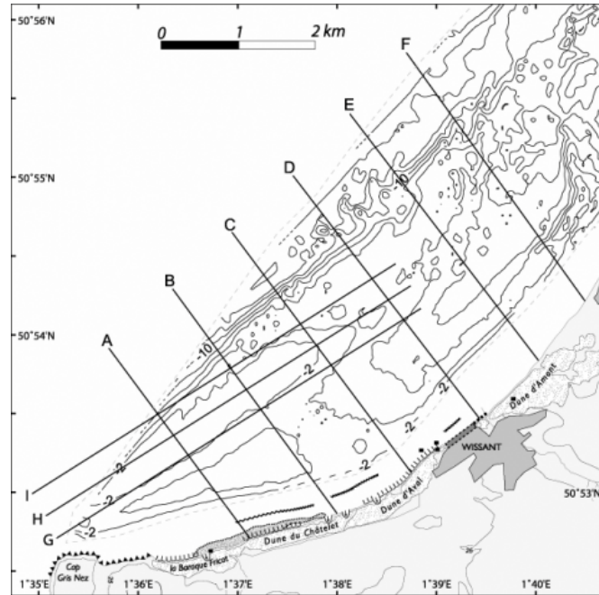
Fig. 4 – Localisation des profils bathymétriques (pour la légende, voir la fig. 1).
