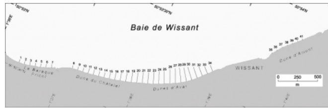
Fig. 2 – Localisation des mesures de position du trait de côte. Fig. 2 – Location of shoreline position measurements.
