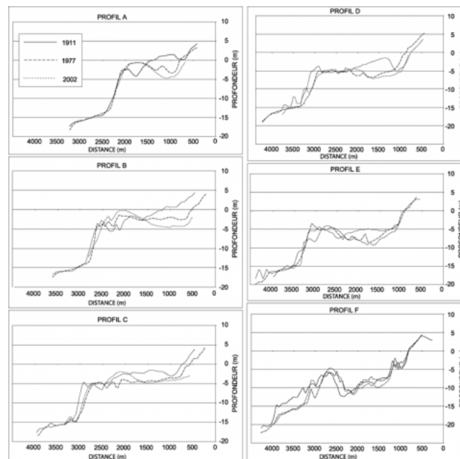
Fig. 8 – Evolution des profils bathymétriques transversaux de 1911 à 2002
