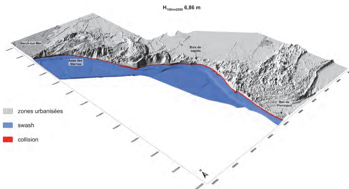
Fig. a-283: Cartographie de l'aléa de submersion marine pour la rive nord de la baie d'Authie et pour un niveau d'eau à période de retour centennale à run-up modéré, à l'horizon 2050 ( H_{100rm2050} ) de 6,86 m IGN69.
