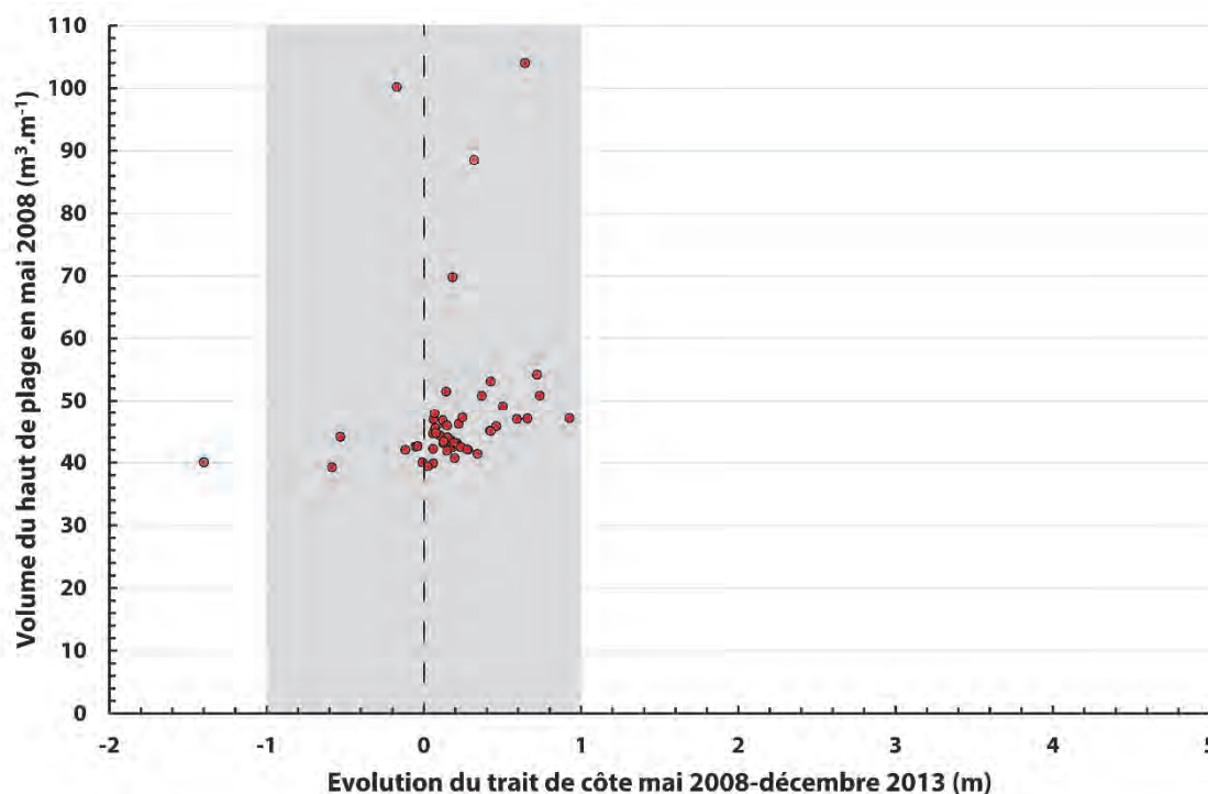
Fig. IV-177 : Evolution du trait de côte entre 2008 et 2013 du littoral allant de Equihen-Plage à Hardelot- Plage en fonction du volume initial (2008) du haut de plage. Le Plancher est à 0,805 m IGN 69 pour les volumes.
