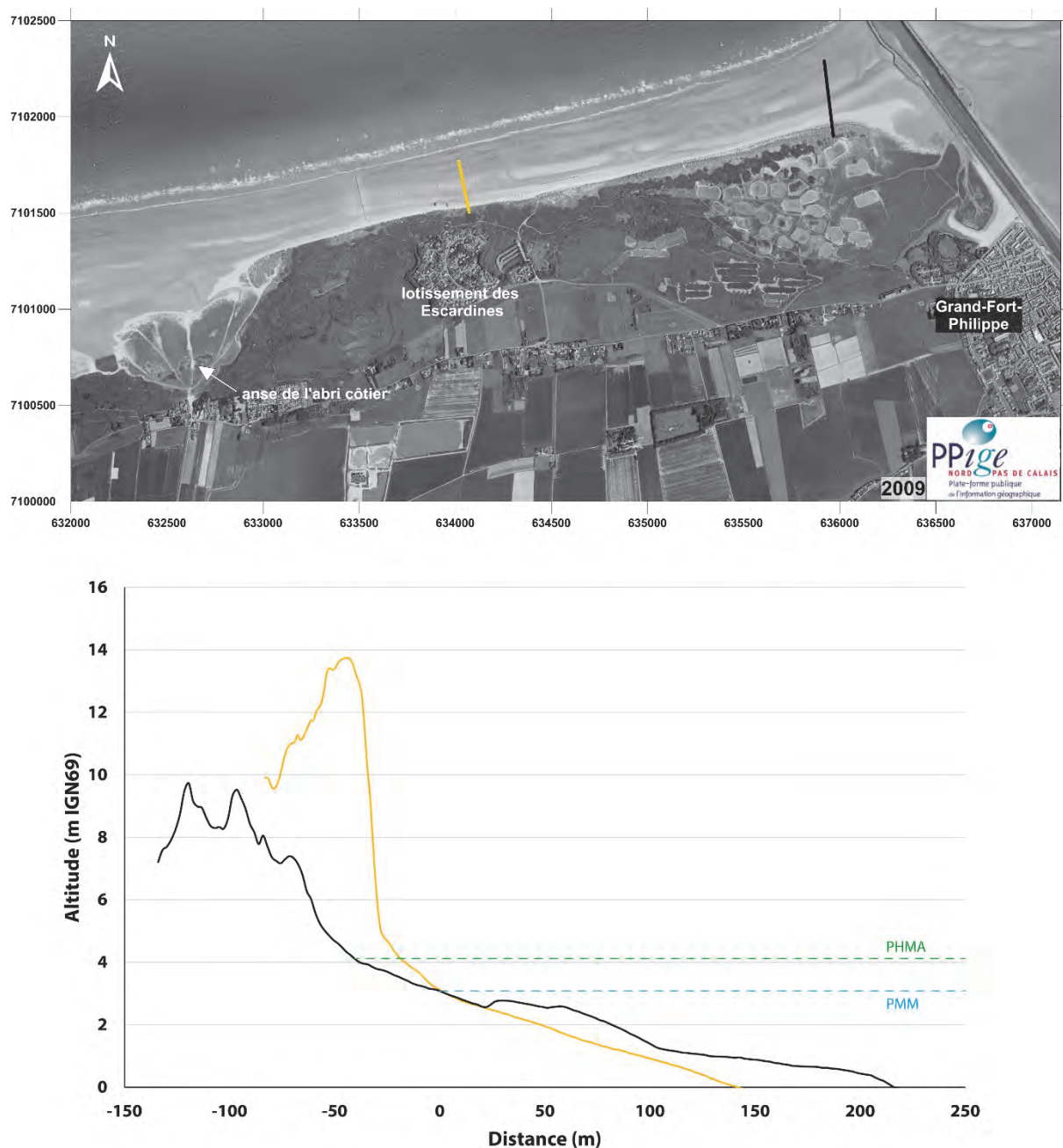
Fig. IV-216: Profils topographiques du massif dunaire du Platier d'Oye illustrant le lien entre la largeur du haut de plage et l'évolution du trait de côte.
