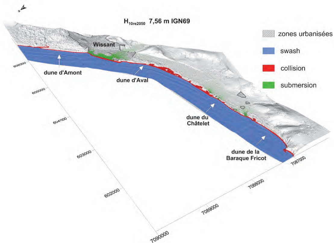
Fig. a-275: Cartographie de l'aléa de submersion marine pour la baie de Wissant et pour un niveau d'eau à période de retour décennale à run-up extrême, à l'horizon 2050 ( H_{10re} ) de 7,56 m IGN69.
