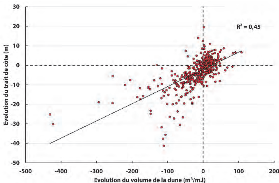
Fig. IV-192 : Evolution du trait de côte et des volumes des dunes de mai 2008 à janvier 2014 en Baie de Wissant.
