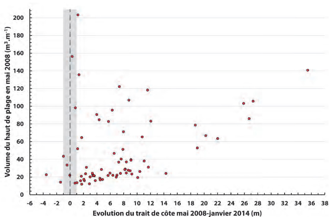
Fig. IV-203 : Evolution du trait de côte entre 2008 et 2014 du littoral allant de Sangatte à Calais en fonction du volume initial (2008) du haut de plage.
