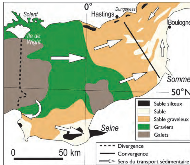
Fig. I-16 : Couverture superficielle sédimentaire de la Manche (Anthony, 2002).
