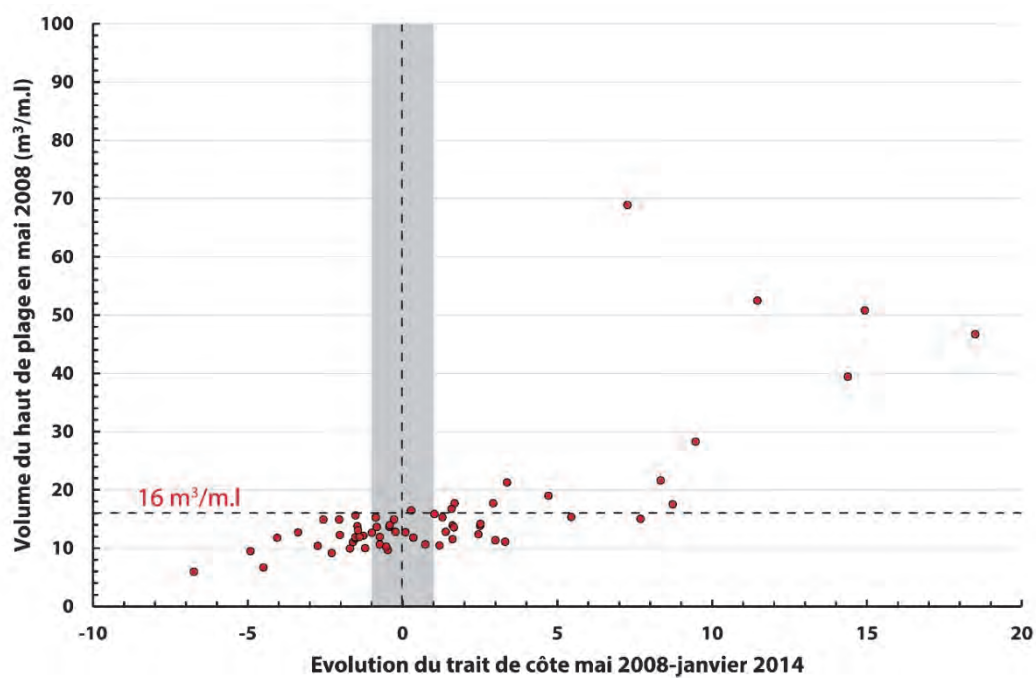
Fig. IV-214 : Evolution du trait de côte entre 2008 et 2014 du littoral du Platier d'Oye en fonction du volume initial (2008) du haut de plage. Le Plancher est à 0,249 m IGN 69 pour les volumes.
