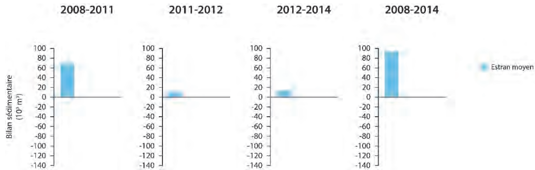
Fig. IV-186: illustration des bilans sédimentaires de la plage de Strouanne.
