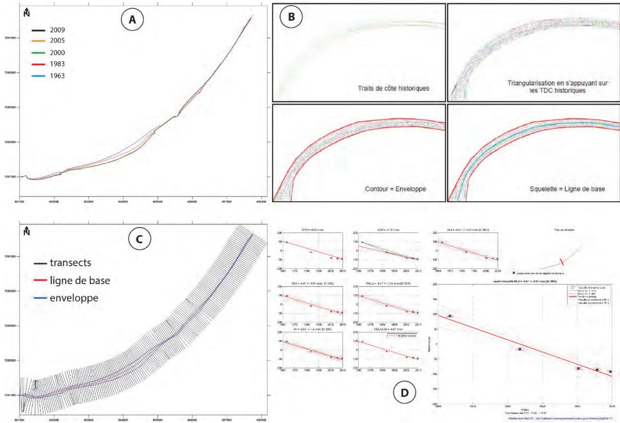
Fig. II-21 : Étapes de calcul de l'évolution du trait de côte : A : digitalisation des traits de côtes à partir de photographies aériennes ortho-rectifiées et géo-référencées. B : création de la ligne de base par squelettisation. C : illustration de l'enveloppe, la ligne de base et les transects sur le secteur de la baie de Wissant. D : paramètres statistiques de l'évolution du trait de côte calculés pour un transect de la baie de Wissant.
