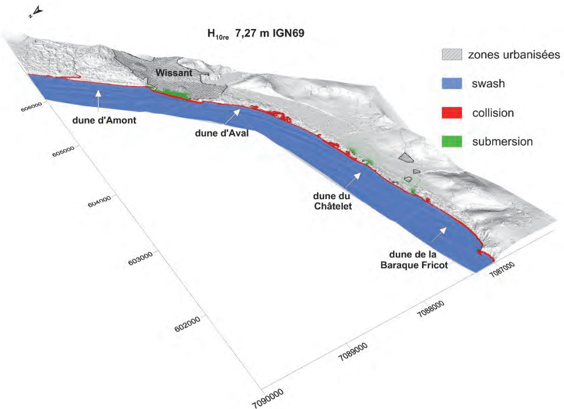
Fig. a-274: Cartographie de l'aléa de submersion marine pour la baie de Wissant et pour un niveau d'eau à période de retour décennale à run-up extrême ( H_{10re} ) de 7,27 m IGN69.
