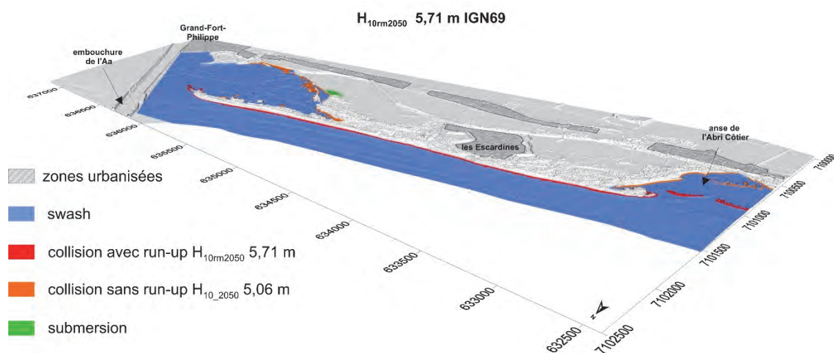
Figure 267: Cartographie de l'aléa de submersion marine pour le secteur littoral du Platier d'Oye et pour un niveau d'eau à période de retour décennale à run-up modéré, à l'horizon 2050 ( H_{10rm\ 2050} ) de 5,71 m IGN69.
