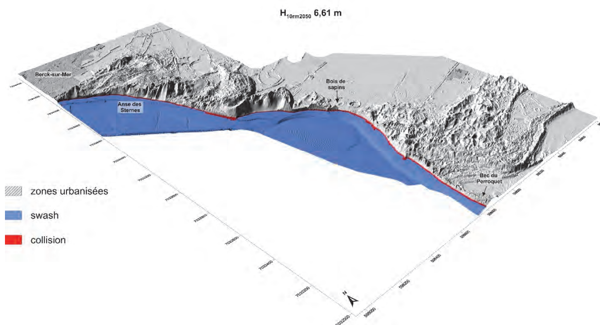
Fig. a-279: Cartographie de l'aléa de submersion marine pour la rive nord de la baie d'Authie et pour un niveau d'eau à période de retour décennale à run-up modéré, à l'horizon 2050 ( H_{10m2050} ) de 6,51m IGN69.
