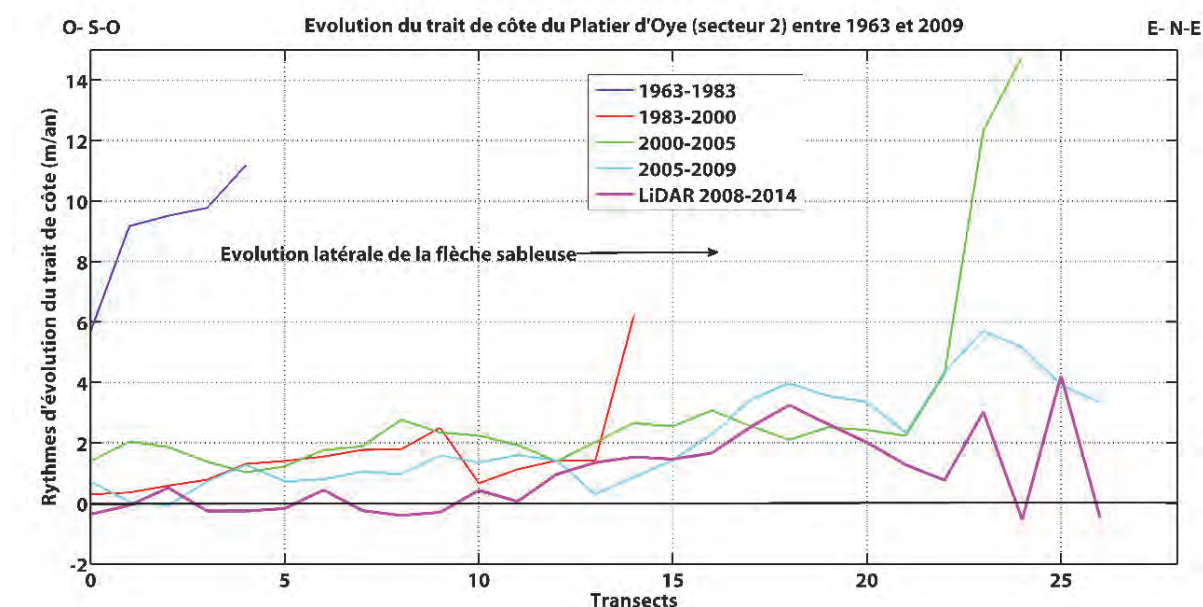
Fig. III-116 : Evolution du trait de côte du Platier d'Oye (secteur 2) entre 1963 et 2009 et entre 2008 et 2014 (LiDAR).
