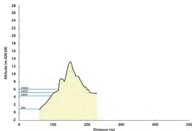
Fig. III-59 : Coupe topographique du cordon dunaire au niveau du Bec du Perroquet, issue des données LiDAR de décembre 2013. PHMA : niveau des plus hautes mers astronomiques, PMM : niveau des pleines mers moyennes, NM : niveau moyen de la mer.
