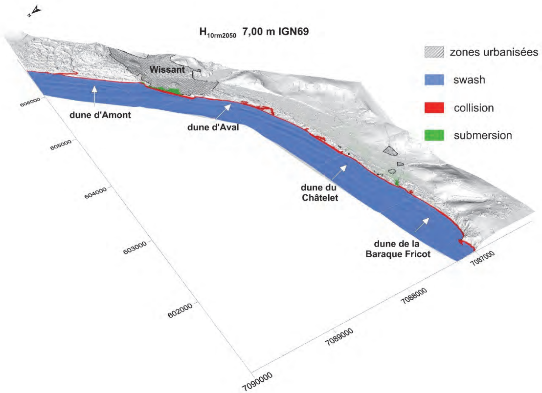
Fig. a-273: Cartographie de l'aléa de submersion marine pour la baie de Wissant et pour un niveau d'eau à période de retour décennale à run-up modéré, à l'horizon 2050 ( H_{10m2050} ) de 7,00 m IGN69.
