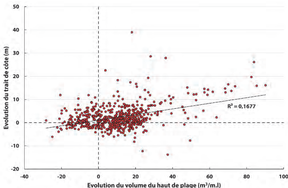
Fig. IV-161 : Evolution du trait de côte et des volumes du haut de plage de mai 2008 à décembre 2013 sur le littoral s'étendant de Berck-sur-Mer au Touquet-Paris-Plage.
